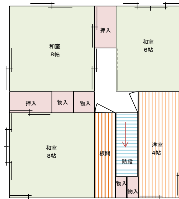
2階平面図
